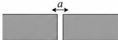
单缝衍射
