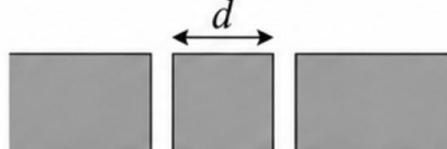
双缝衍射
